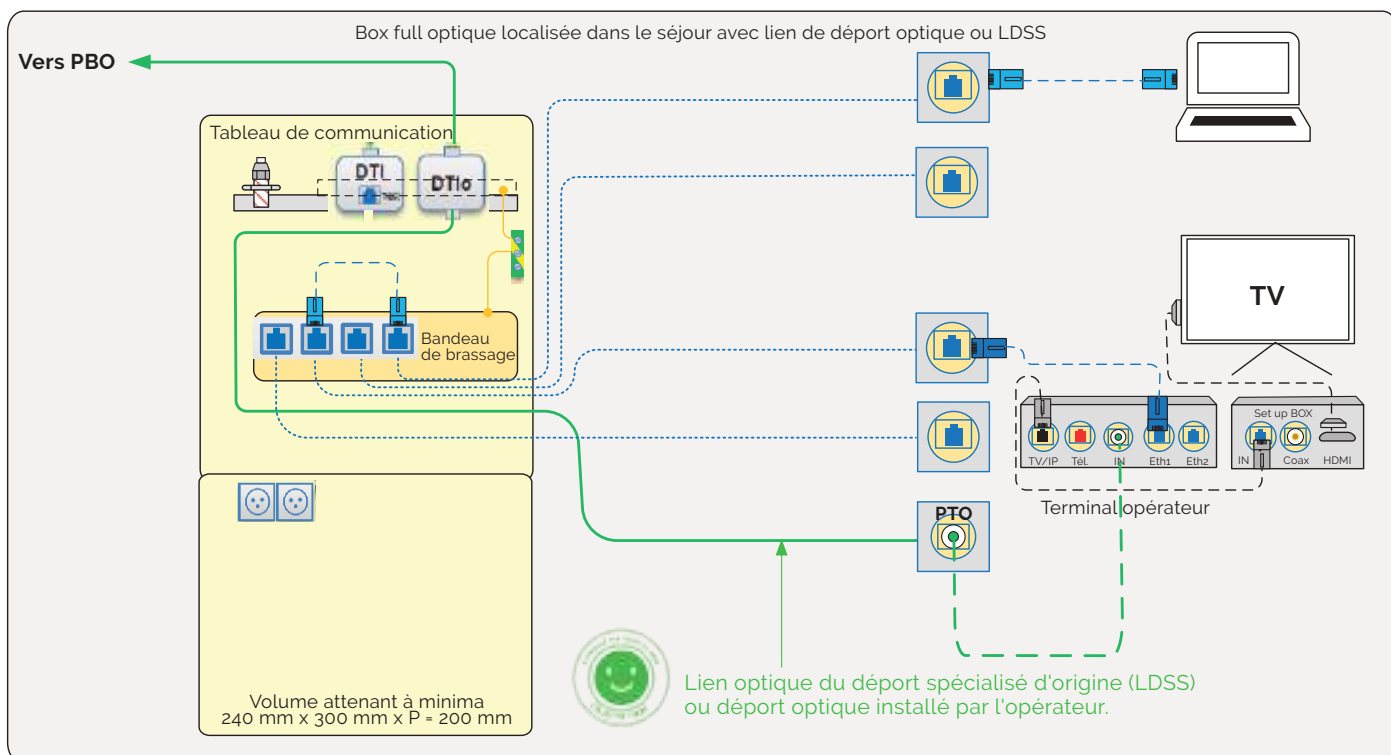
Fig. 75 | Distribution du logement avec une box full optique localisée dans le séjour et lien de dépôt optique
