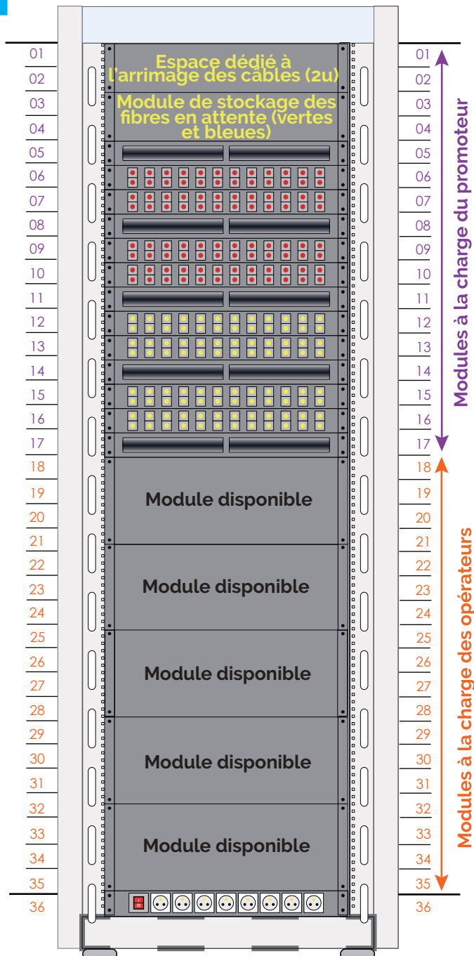
Fig. 42 | Exemple de love de câble de la colonne de communication en sortie d'un PR
