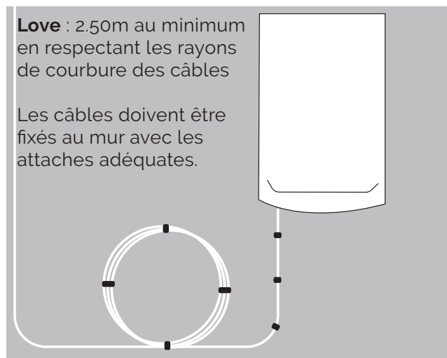
Fig. 42 | Exemple de love de câble de la colonne de communication en sortie d'un PR
