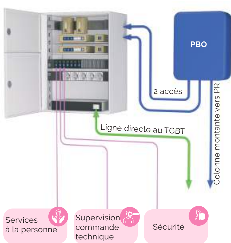
Fig. 66 | Synoptique des différents branchements du coffret de services
